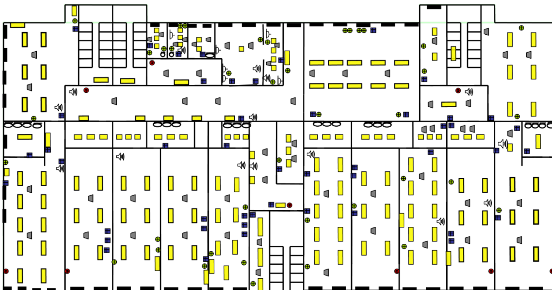
Поэтажный план здания МАДОУ города Нижневартовска ДС № 77 «Эрудит», расположенного по адресу ул.Интернациональная 45 А. (2 этаж)
